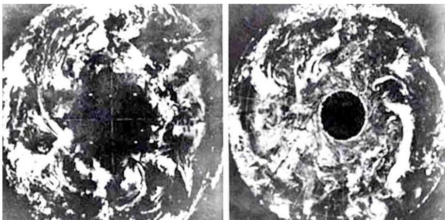
Die linke Aufnahme wurde am 1. Januar 1967 vom ESSA-Satellit aufgenommen, die rechte Aufnahme am 23. November 1968 vom Satelliten ESSA 8. Laut NASA soll es sich um klimatisch bedingte offene Stellen im Meereseis handeln.
