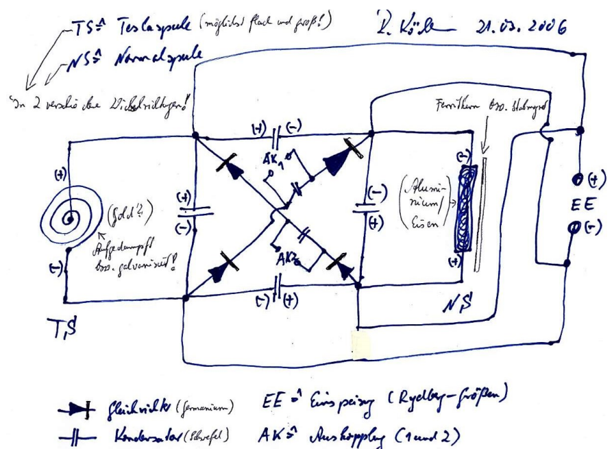
Rudimentäre Zeichnung der Schaltung von Reinhard Köcher von 2006. Diese wird jetzt durch Jörg Wochian in Zeichnungen mit dem CAD-System umgesetzt.
